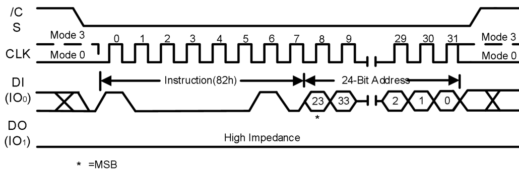
Figure15. Mini Sector Erase Sequence Diagram
